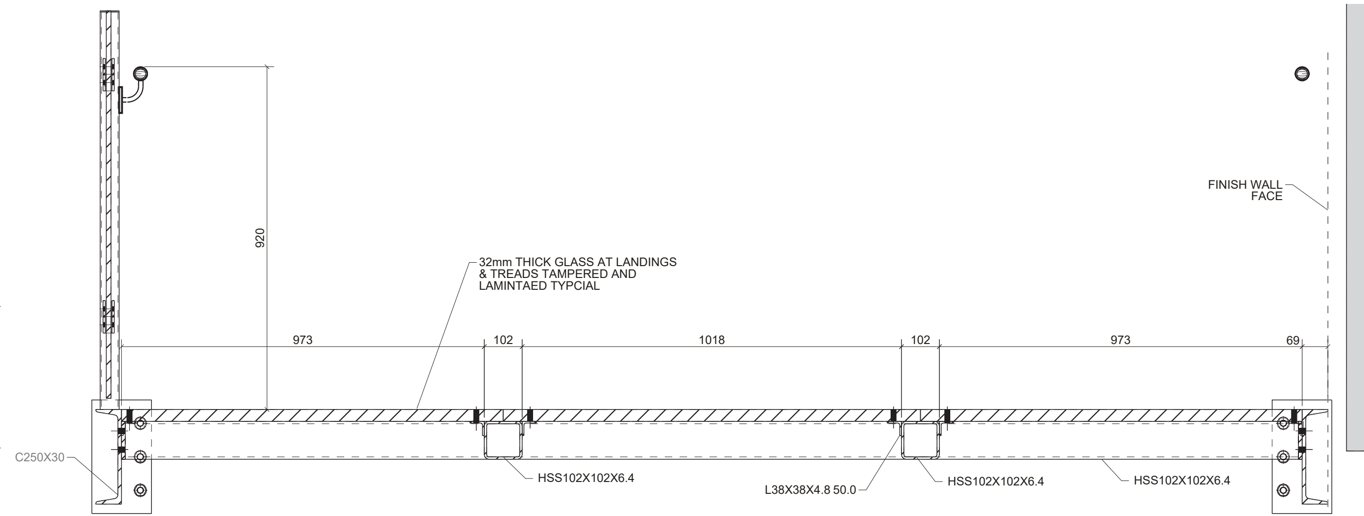
SECTION A-A
