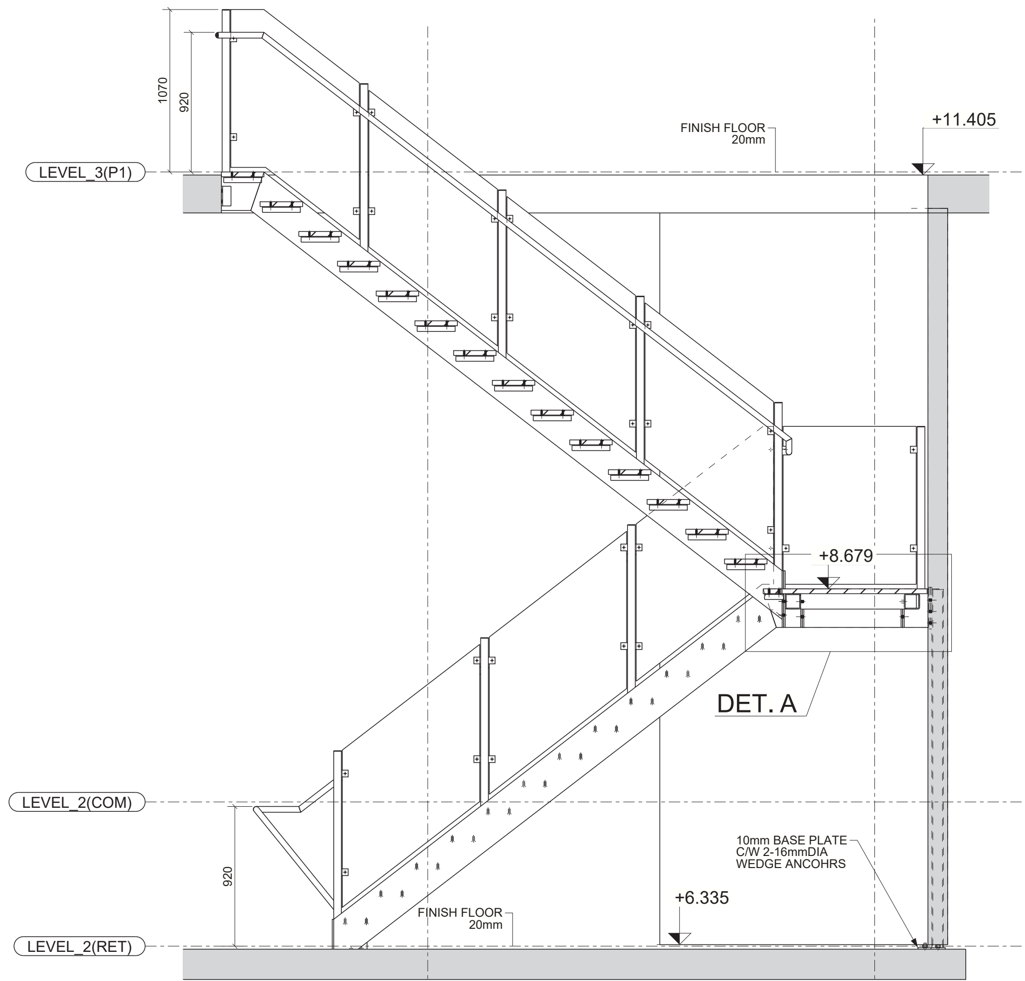
SECTION D-D E01
